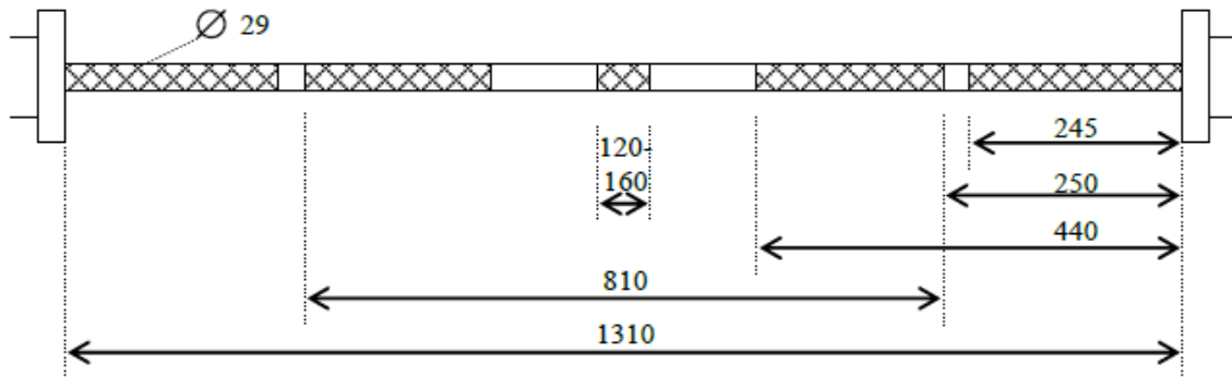
Размеры в мм (насечка между втулками)
